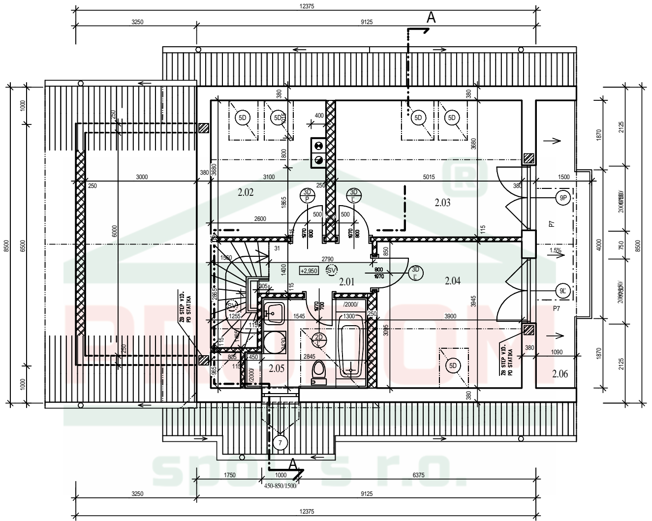
PREMIER 93 - Z0 - 2.NP
