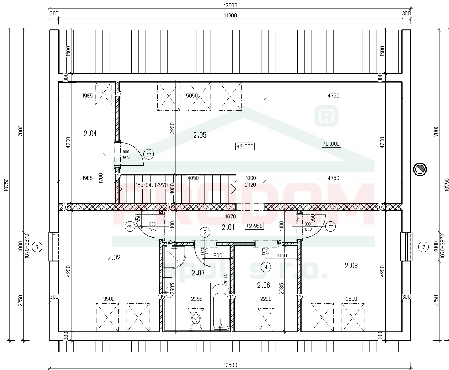
MERKUR 2 - 2.NP - ZO
