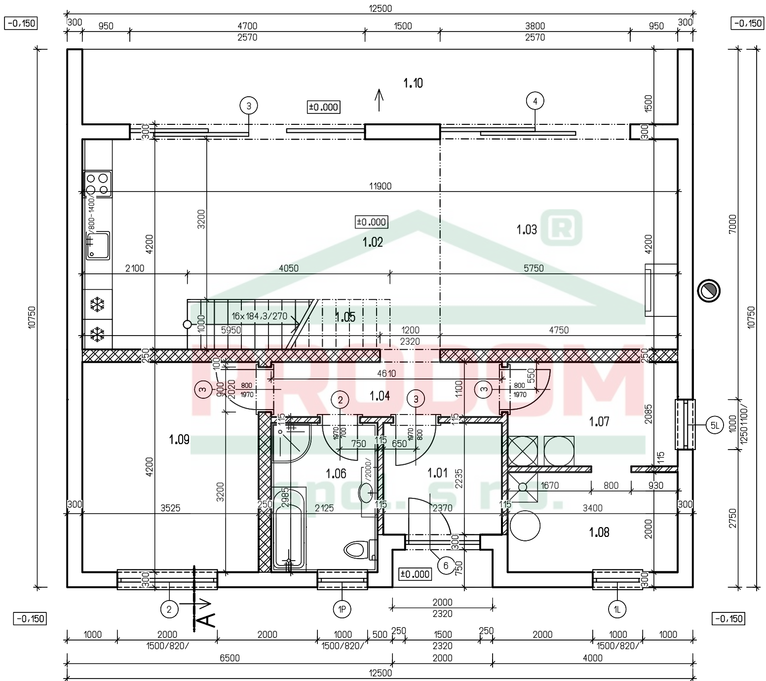
MERKUR 2 - 1.NP - ZO
