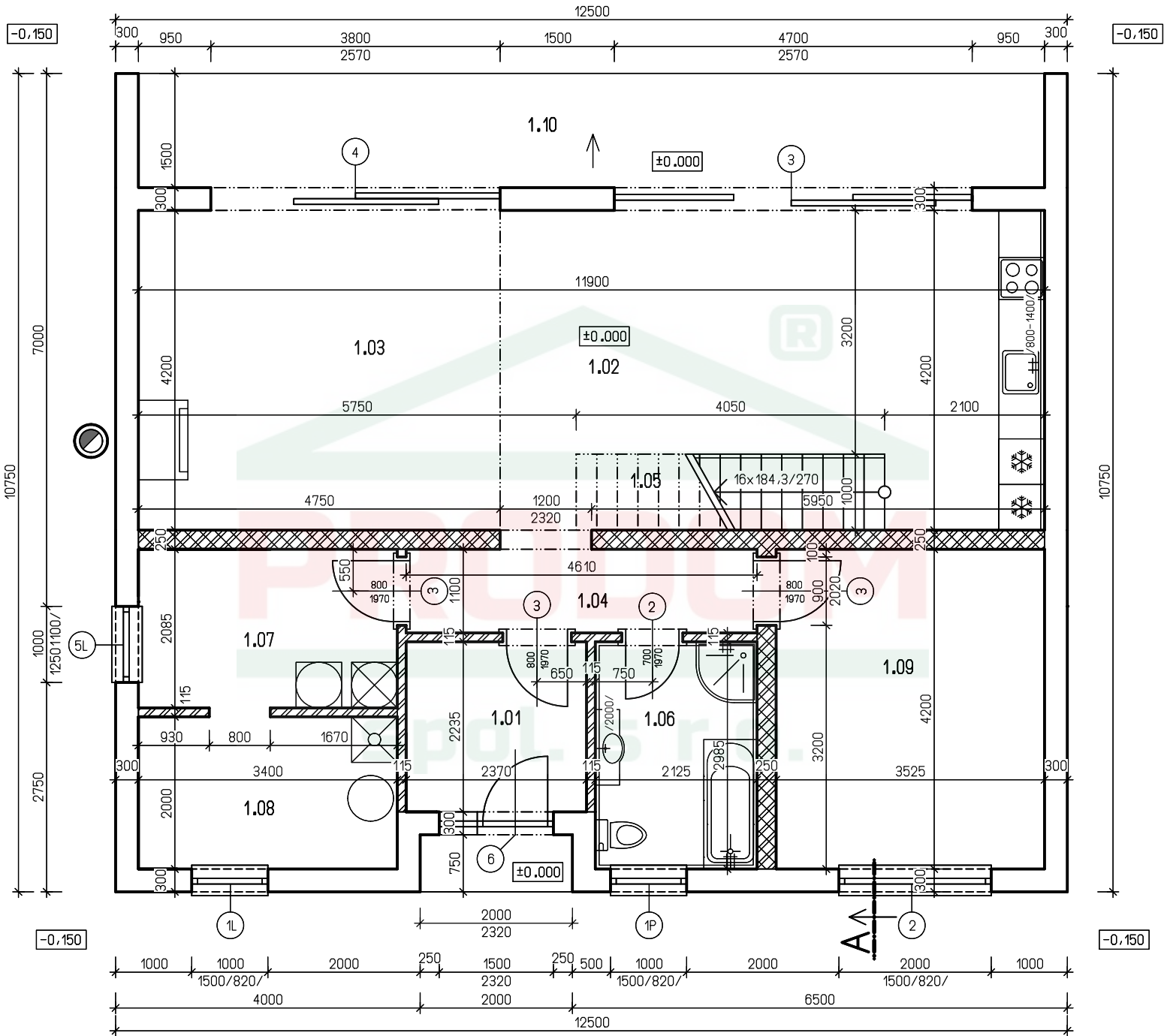
MERKUR 2 - 1.NP
