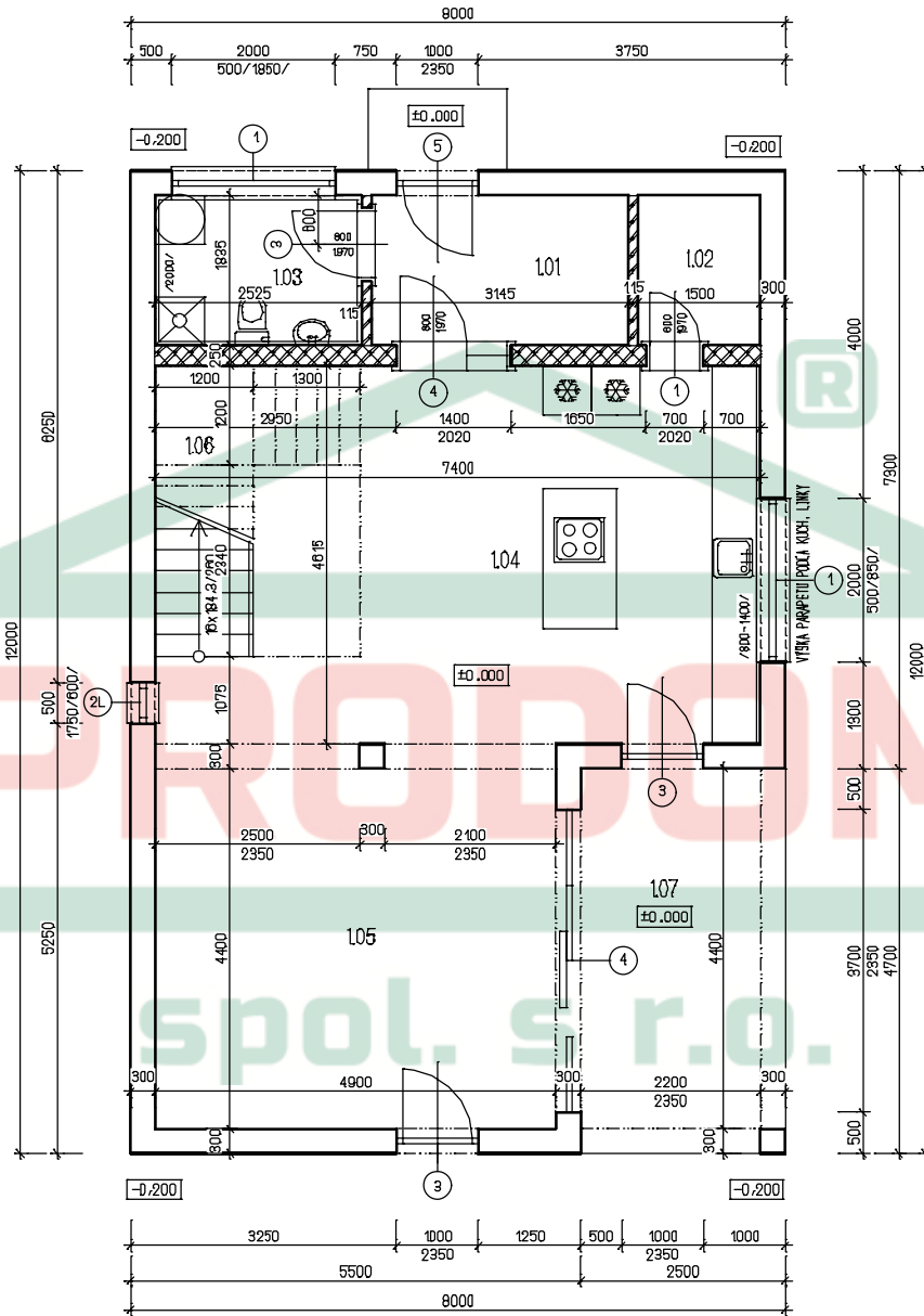
ARKADA 14 - 1.NP - Z0
