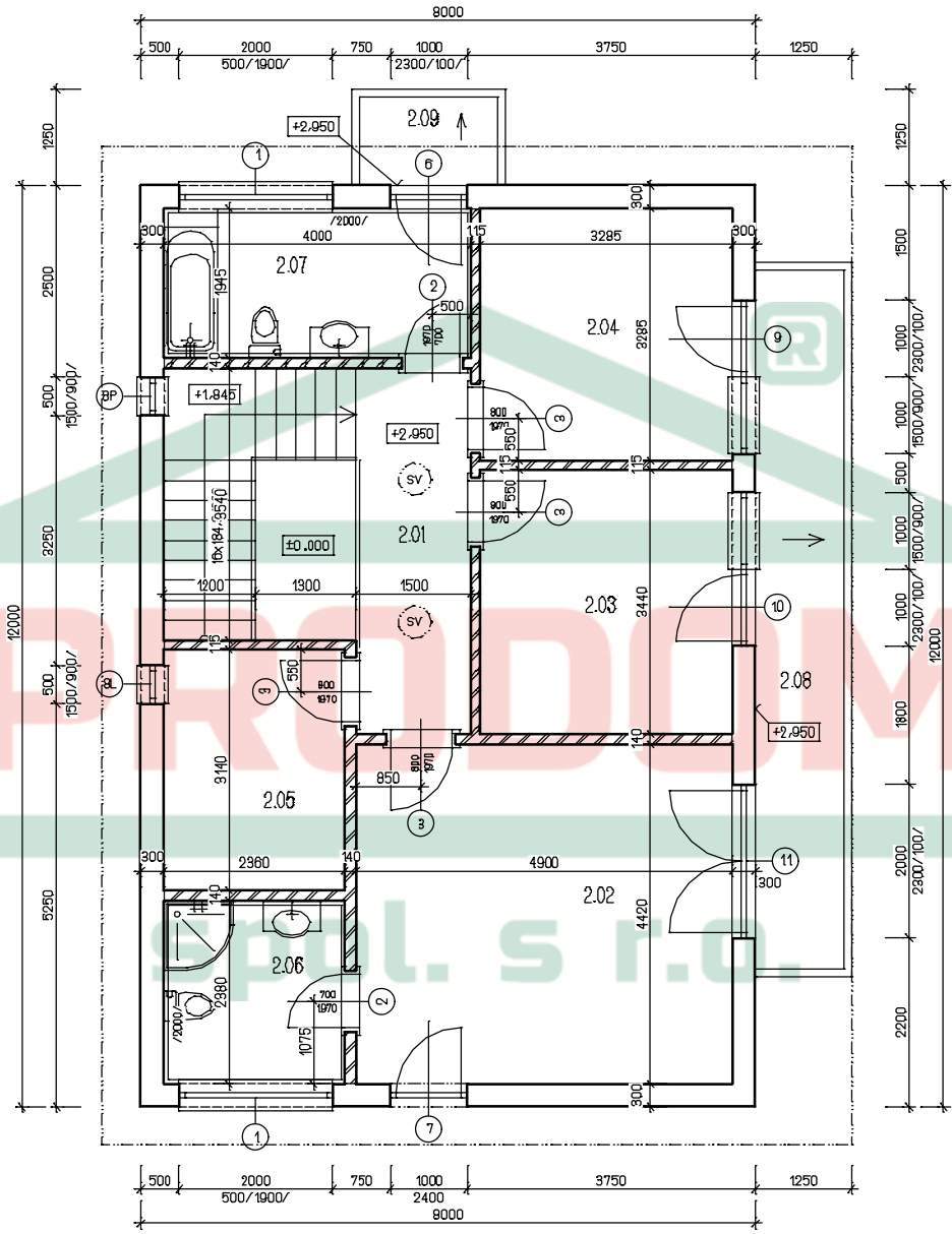
ARKADA 14 - 2.NP - Z0
