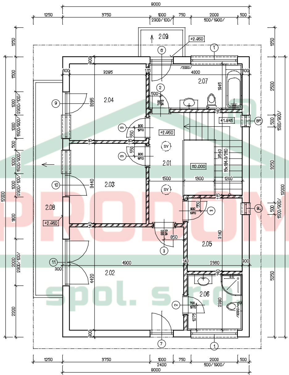
ARKADA 14 - 2.NP
